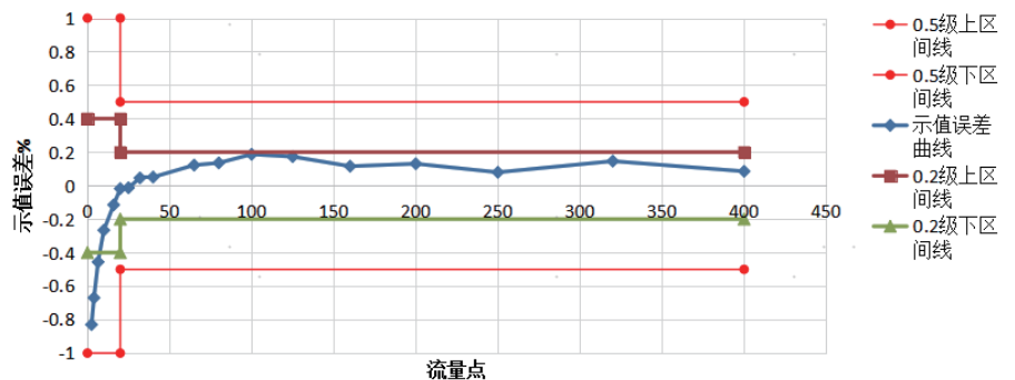
G250 规格流量计示值误差曲线
